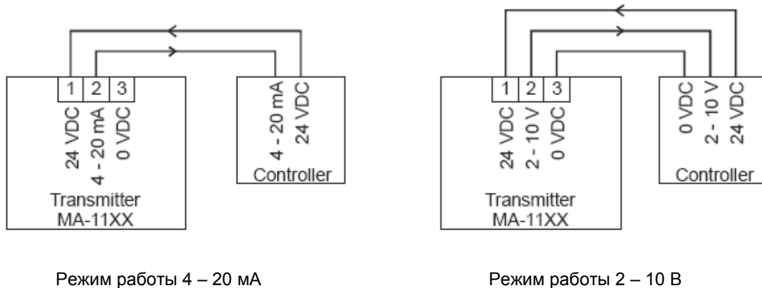
Рис. 2 Диаграмма кабелей
