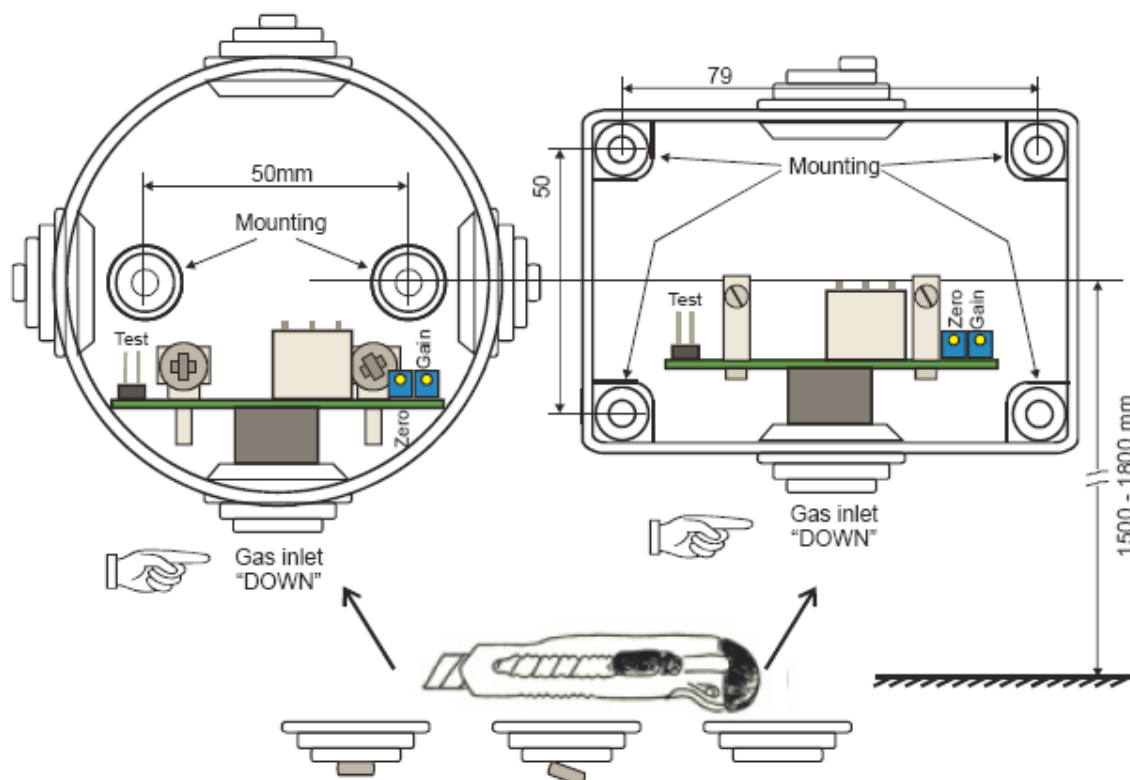
Рис. 1. Монтаж устройства.
