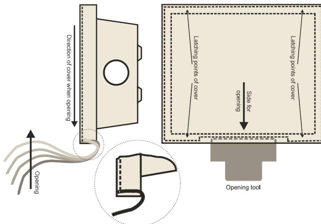
Рис. 10 Вскрытие корпуса типа 5
