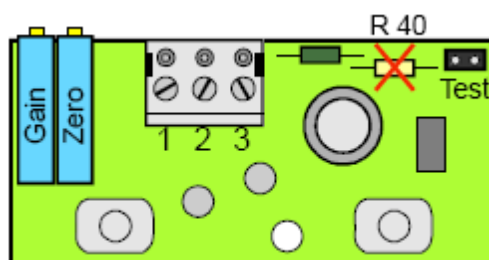
Рис. 4 Основная плата
