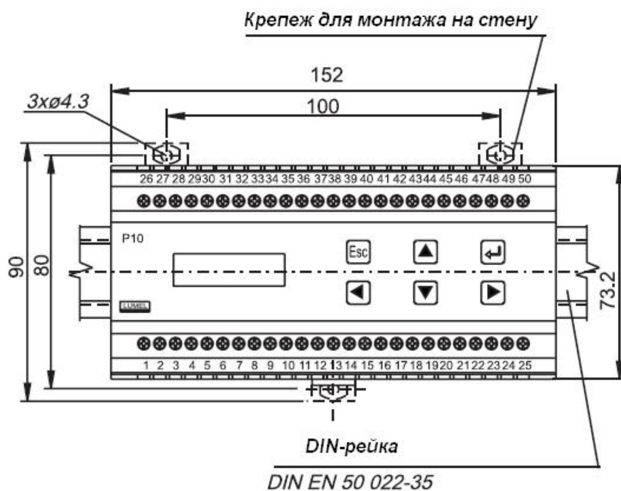
Рис.1. Габариты и способ монтажа прибора
