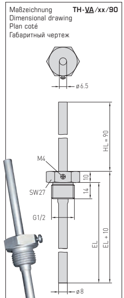
TH-VA/xx/90 Edelstahhtauchhülse mit Halsrohr Stainless steel immersion sleeve with neck tube doigt de gant en acier inox avec tube prolongateur Гильза погружная из высококачественной стали с горловиной
