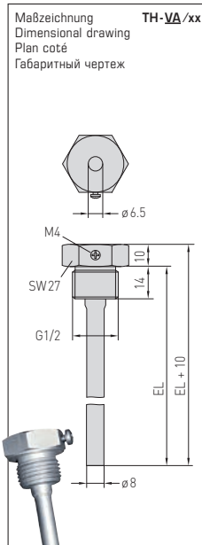
TH-VA/xx Edelstahhtauchhülse Stainless steel immersion sleeve doigt de gant en acier inox Гильза погружная из высококачественной стали
