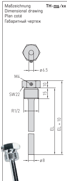
TH-ms/xx Messingtauchhülse Brass immersion sleeve doigt de gant en laiton Гильза погружная из латуни
