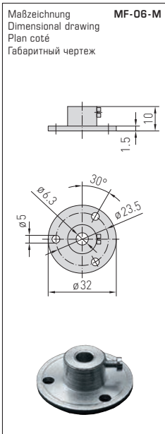
MF-06-M Montageflansch aus Metall Mounting flange, metal Bride de montage en métal Присоединительный фланец из металла
