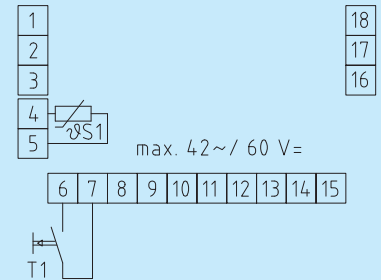
Схема соединения
